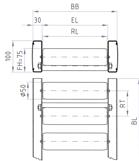
Tragrollen in mittlerer Lochreihe montiert
