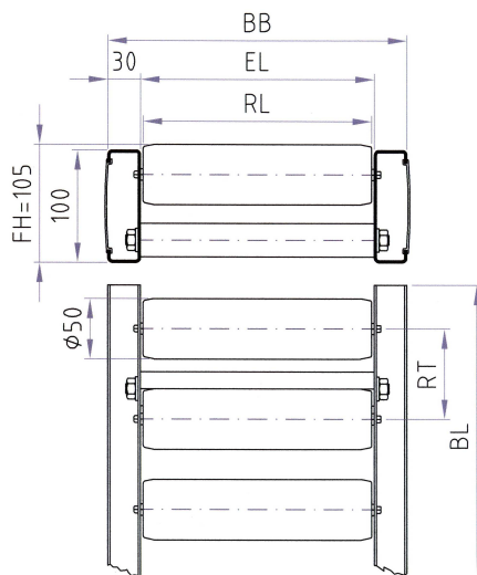
Tragrollen in oberer Lochreihe montiert
