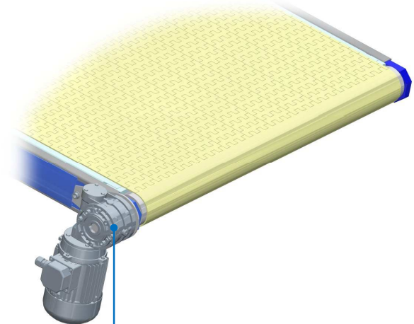
Ausführung Getriebemotor aufgesteckt
