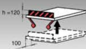
Abrollsicherung
