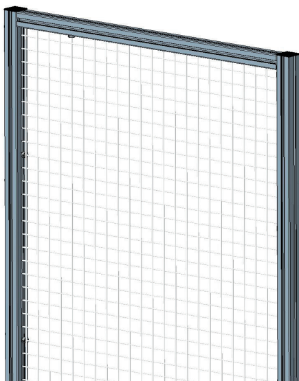
Füllung: Wellgitter 40x40 mm verzinkt
